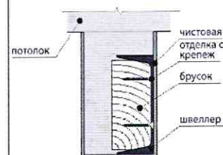
Конструкция внутри проема
